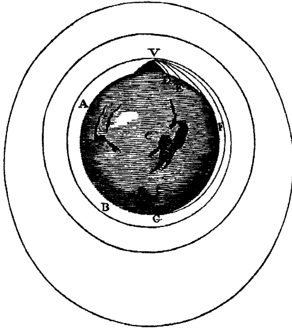
رسمٌ توضيحي من كتاب المبادئ لنيوتن يمثل قذيفةً في مسارها حول الأرض.
